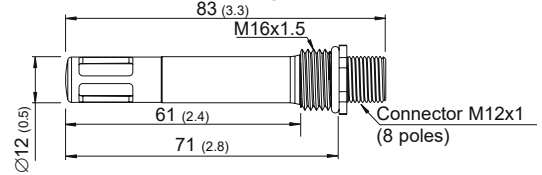
EE08 with connector (Type E11)
